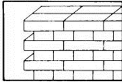
Fig. 26 A sogá y tizón inglés.
