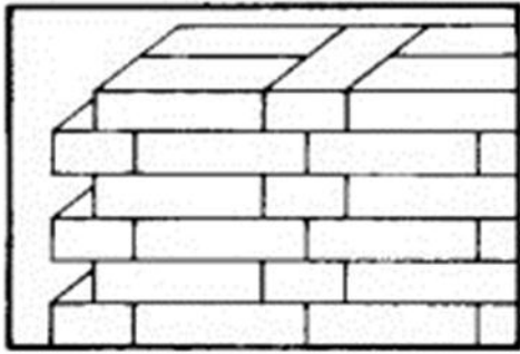
Fig. 25 A sogá y tizón diatónico.
