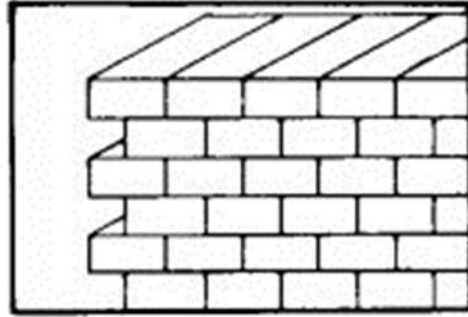
Fig. 23 A tizón. Tb. de llaves, de asta.
