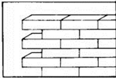
Fig. 24 A sogá. Tb. de cítara, de media asta.
